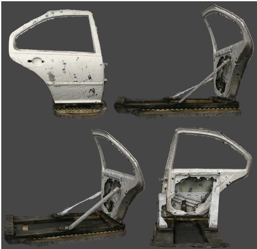
Figura 74.1: Reconstrucción digital de una puerta de automóvil perforada por proyectiles de arma de fuego. Imagen del autor y E. Bárcenas Hernández (qepd).
