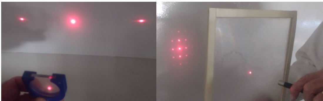
Figura 6.1. Patrones de difracción producidos con un láser cuando pasa por A) un cabello; B) una rejilla múltiple vertical y C) una rejilla múltiple cuadriculada (elaboración propia).
