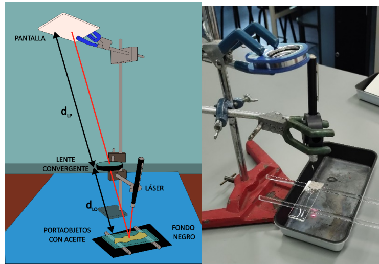
Figura 7.5. Arreglo experimental. A la izquierda, esquema del arreglo; y a la derecha, detalle de colocación del láser, la muestra y el lente (elaboración propia).
