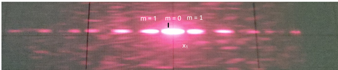
Figura 5.10. Patrón de interferencia producido al pasar el láser por una doble rendija. Se señalan las dos bandas laterales luminosas de orden m = 1 , que en este caso son las únicas que se obtienen en la interferencia de las bandas luminosas centrales (elaboración propia).
