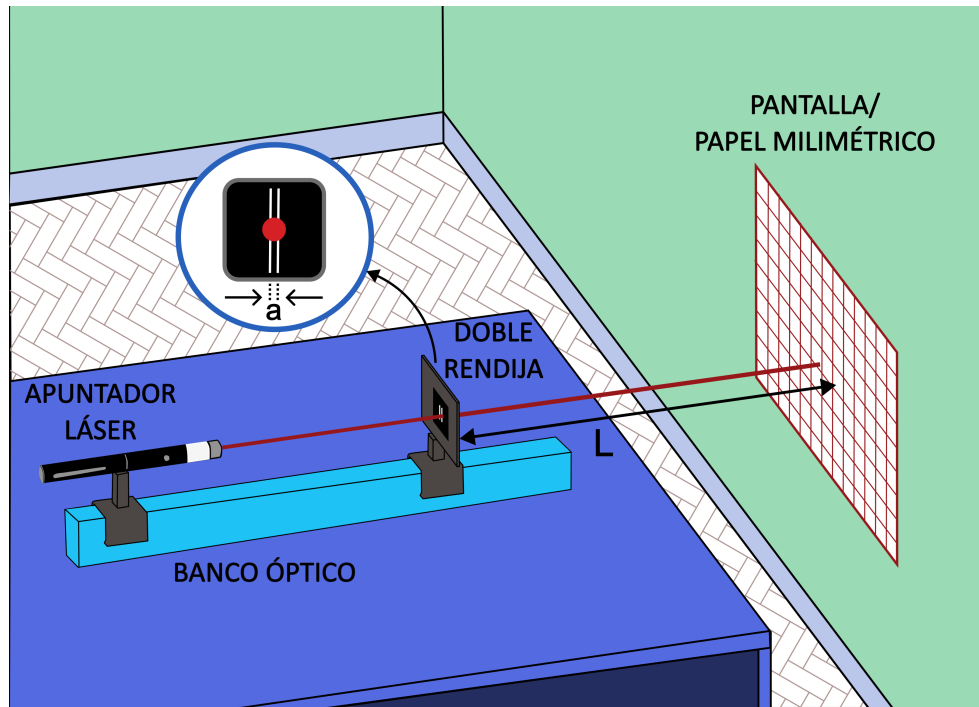
Figura 5.9. Disposición de los elementos experimentales. En el círculo se muestra la doble rendija de frente, el punto rojo ilustra la luz láser incidiendo en las rendijas. Los centros de las rendijas están separados la distancia a (elaboración propia).
