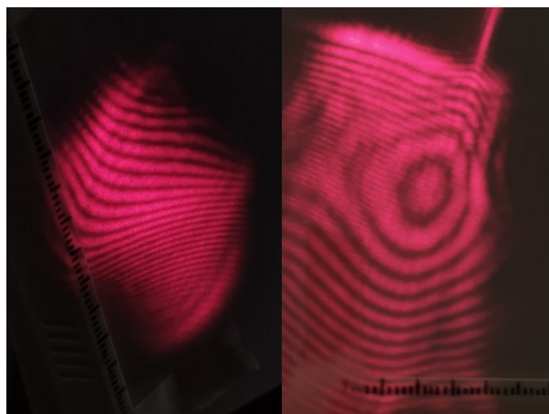
Figura 7.7. Patrones de interferencia. Se observa el patrón de interferencia de la película delgada por diferencia de tamaño y separación de las franjas oscuras y brillantes (elaboración propia).
