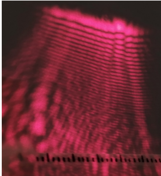
Figura 7.8. Imagen centrada en el patrón de interferencia debido a la película de aceite. Las franjas superiores son más gruesas y brillantes que las inferiores (elaboración propia).
