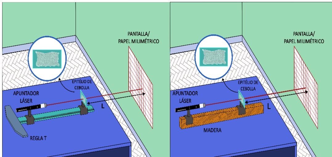
Figura 6.2. Diversas maneras de montar el banco óptico (elaboración propia).
