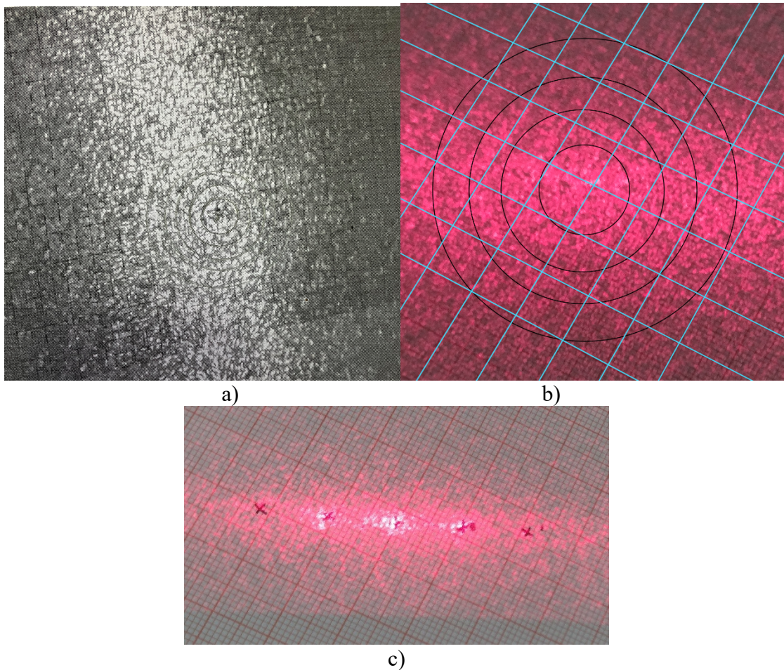
Figura 6.5. Patrones de difracción a) y b) circulares trazados en papel; c) patrón tipo rendija (elaboración propia).
