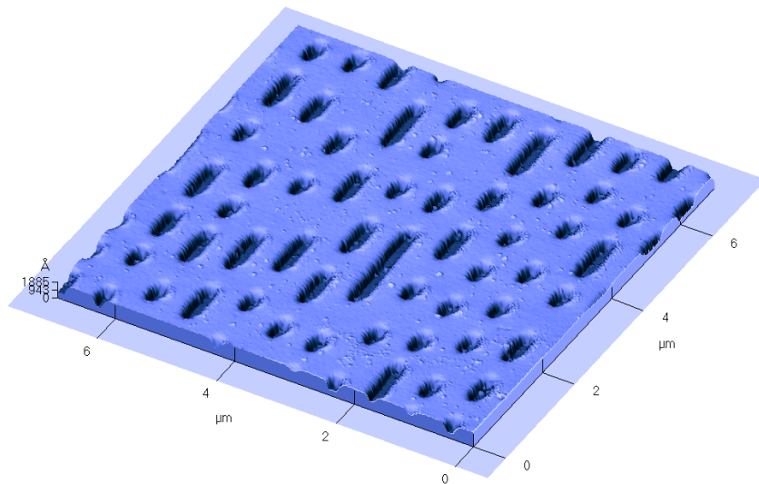
Figura 8.5. Micrografía de un Disco de Video Digital (DVD) obtenida por microscopia de fuerza atómica. La imagen tiene un largo y ancho de 7 \mu\text{m} (cortesía del M. en C. José Guadalupe Bañuelos Muñetón del ICAT).
