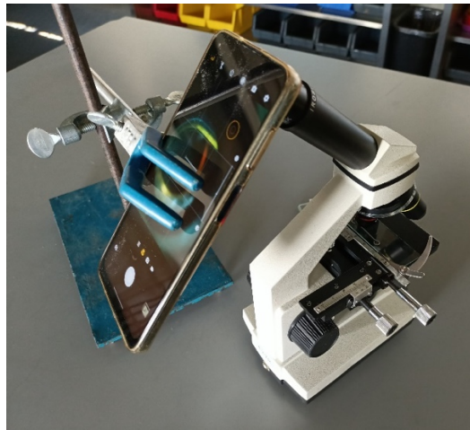
Figura 4.7. Montaje de teléfono celular colocado al frente del ocular para tomar fotografías (elaboración propia).
