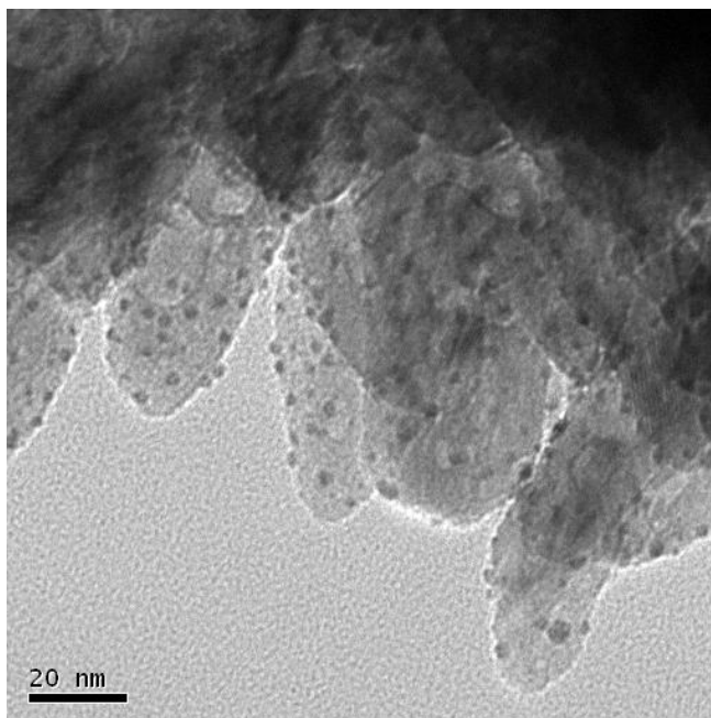
Figura 8.8. Nanopartículas de oro (pequeños gránulos) en soporte de óxido de titanio, tomadas con un microscopio electrónico (cortesía del Dr. Rodolfo Zanella Specia, del ICAT).
