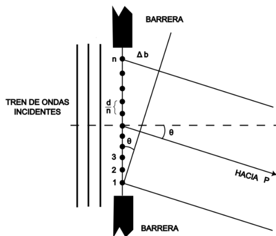
Figura A2.3. Frente de onda producido en dirección P y ángulo \theta (elaboración propia).
