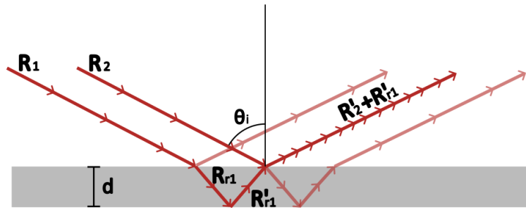
Figura 7.3. Los rayos de luz R_1 y R_2 inciden en la superficie superior de la película delgada. Parte del R_1 se transmite dentro de la película R_{r1} y se refleja en la superficie interior R'_{r1} para salir de la película en el punto donde incide R_2 el cual se refleja parcialmente en la superficie exterior R'_2 . R'_2 + R'_{r1} se superponen, formando el patrón de interferencia de la película delgada (elaboración propia).
