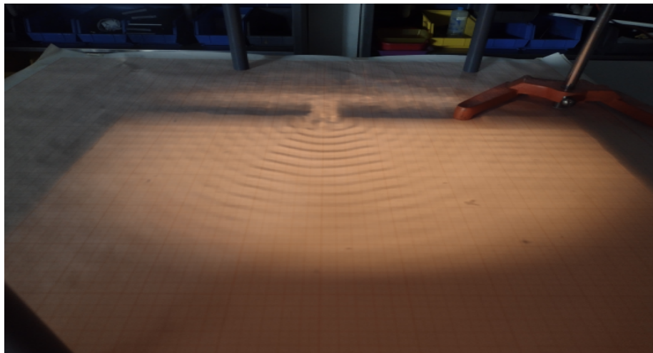
Figura 5.4. Imagen del patrón de difracción producido por una abertura (elaboración propia).
