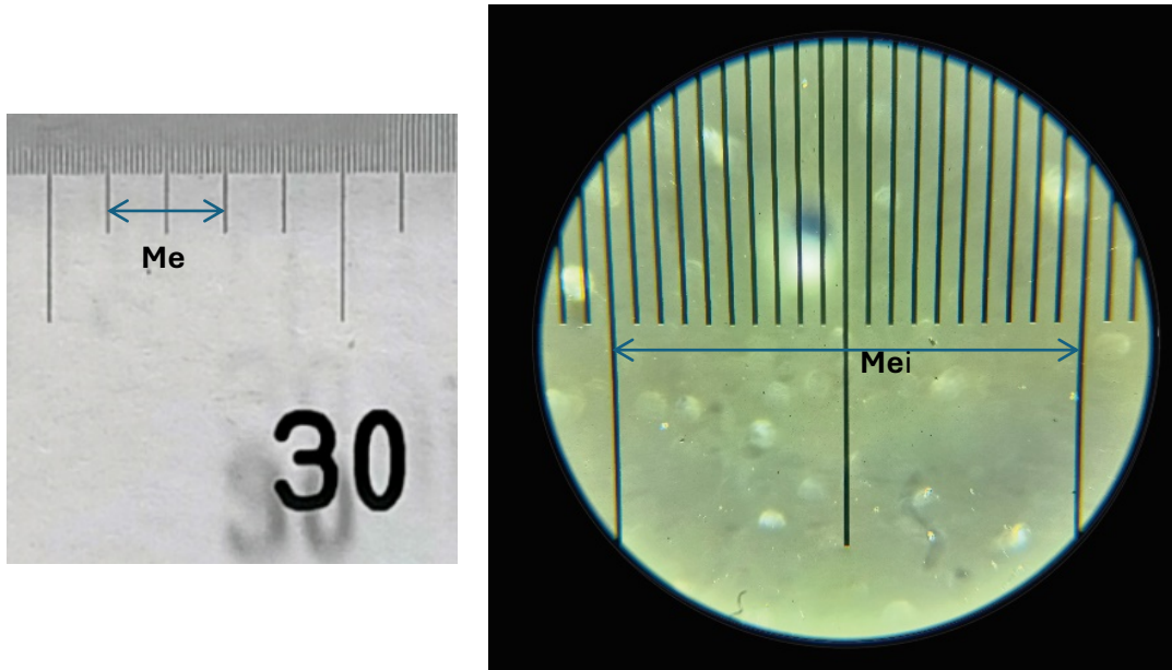
Figura 4.6. Porción de dos milímetros de la regla ( Me ), que se amplifica al proyectar la fotografía tomada cuando se observa a través del microscopio ( Mei ) (elaboración propia).
