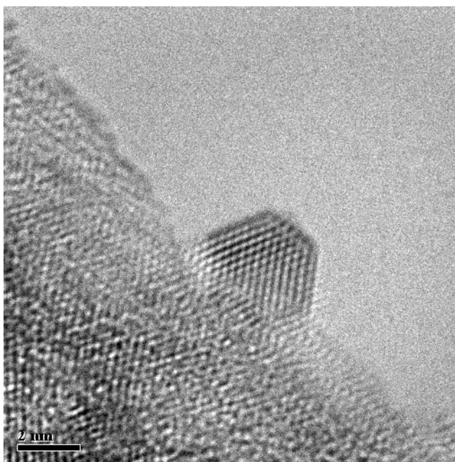
Figura 8.9. En esta imagen (de mayor resolución) se pueden observar los arreglos atómicos de una nanopartícula de oro. Puede distinguirse la forma geométrica (icosaedro) de la nanopartícula y los planos en los que se ordenan los átomos (cortesía del Dr. Rodolfo Zanella Specia, del ICAT).
