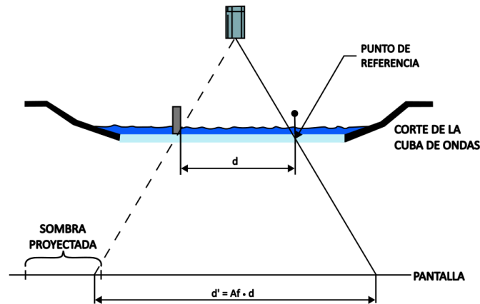
Figura 5.6. Esquema para calcular el factor de amplificación (elaboración propia).
