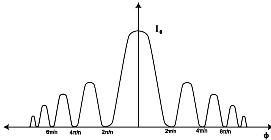
Figura A2.6. Función de intensidad con respecto a la fase (elaboración propia).
