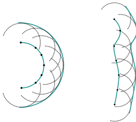
Figura A2.1 Principio de Huygens-Fresnel para diferentes frentes de ondas (elaboración propia).
