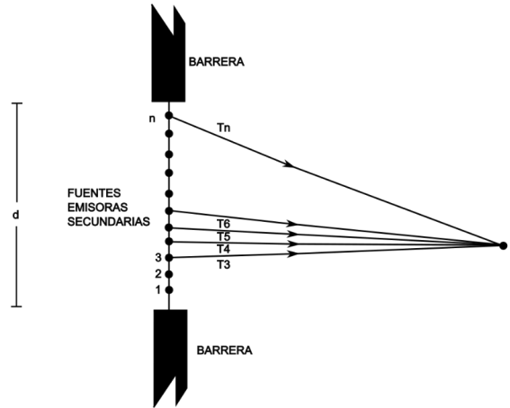
Figura A2.2. Superposición de ondas en un punto P posterior a la abertura (elaboración propia).
