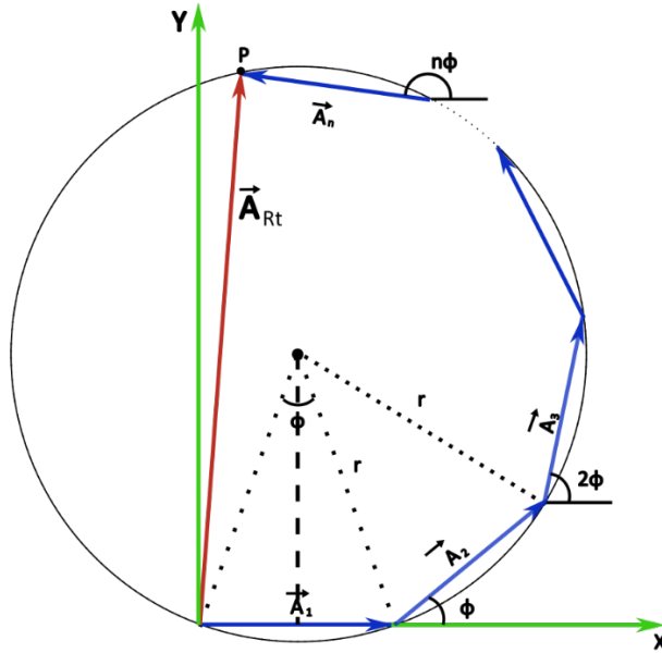
Figura A2.4. Suma vectorial de contribuciones hacia el punto P (elaboración propia).
