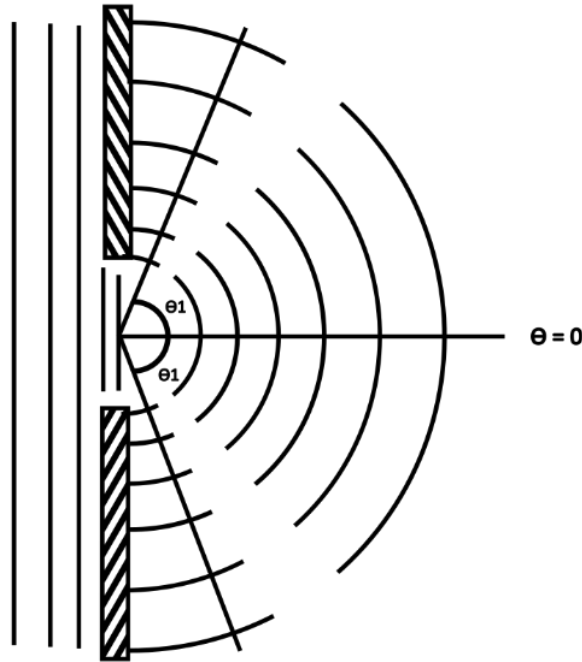
Figura A2.5. Difracción por una rendija (elaboración propia).
