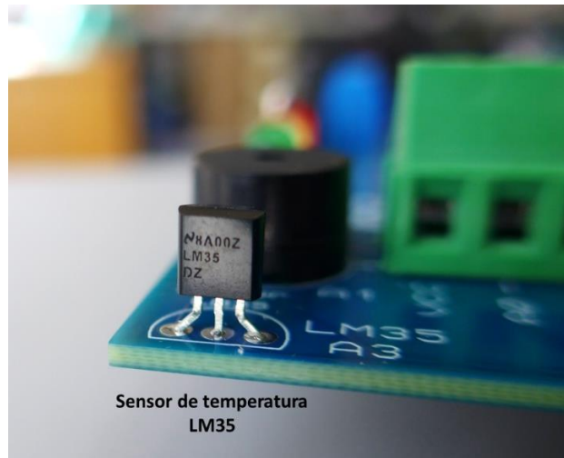
Figura 15. El sensor de temperatura LM35.
