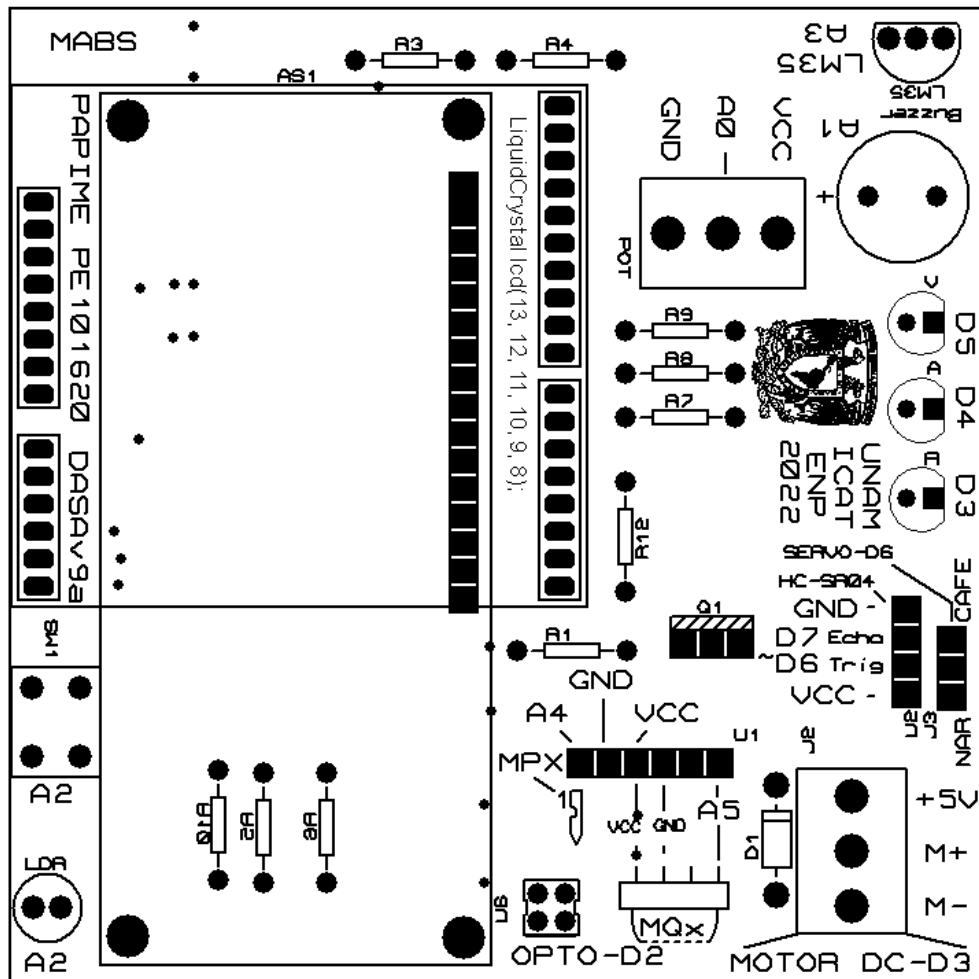
Figura D.1. Serigrafía de la placa del DASA.
