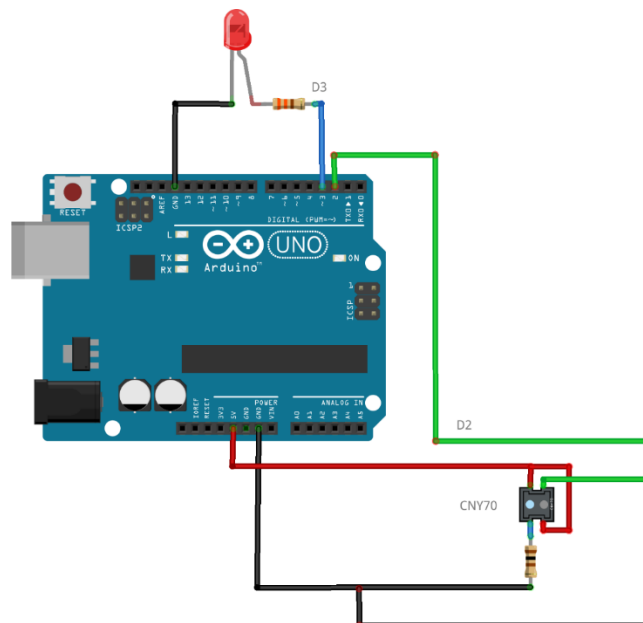
Figura 20. Diagrama de conexiones del optointerruptor CNY70 más un LED.
