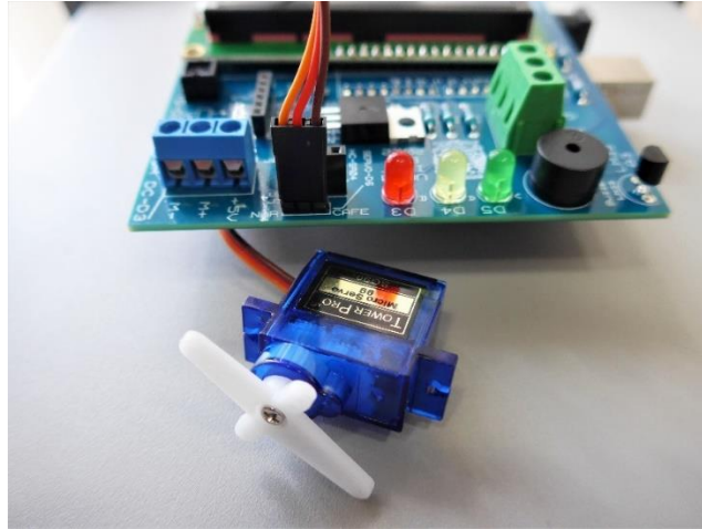
Figura 27. Conexión de un servomotor.
