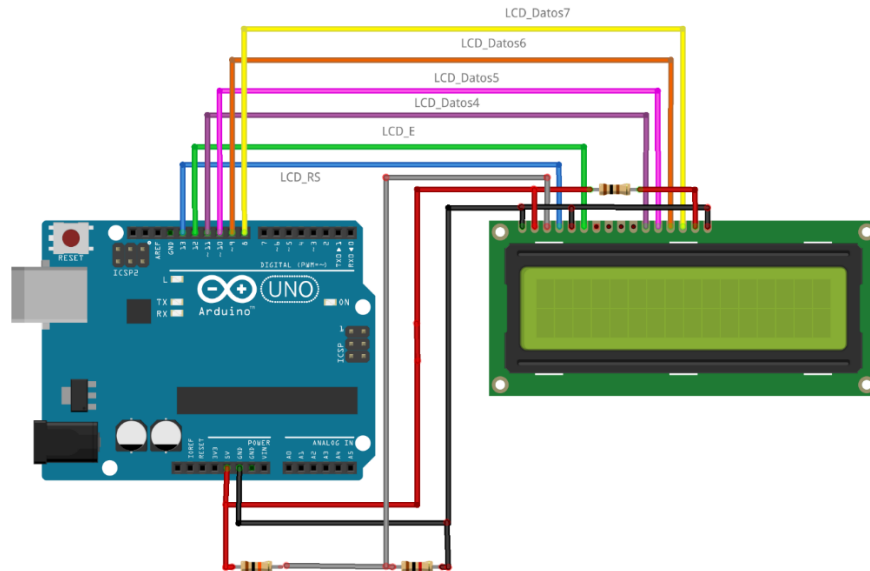
Figura 3. Diagrama de conexiones del display LCD.
