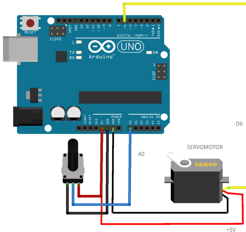
Figura 28. Conexión del servomotor y un potenciómetro.
